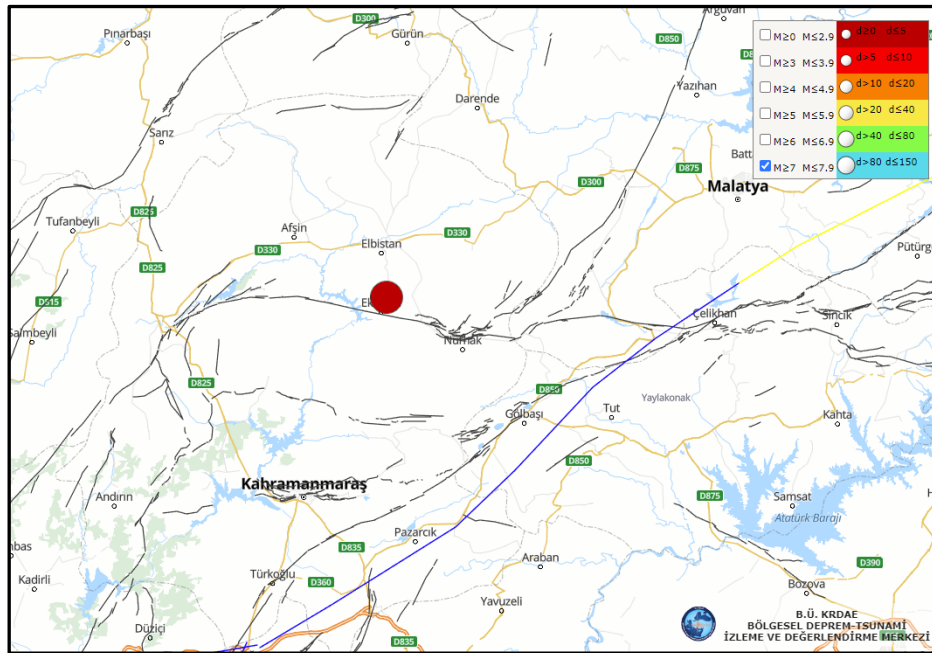
Ekinözü-Kahramanmaraş ( M_l=7.5 ) depreminin lokasyon haritası
